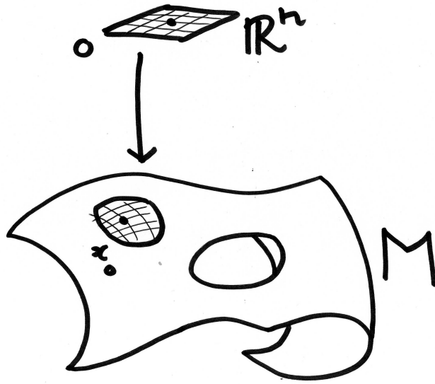
FIG. 4 – Un \mathbf{R}^n -point d'une variété différentielle de dimension n .
